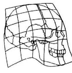
(4) dospělý člověk
