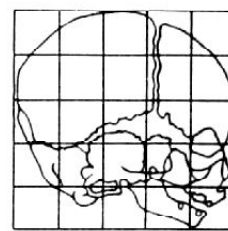
(2) plod člověka
