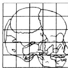
(1) plod šimpanze
