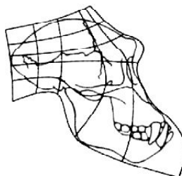
(3) dospělý šimpanz
